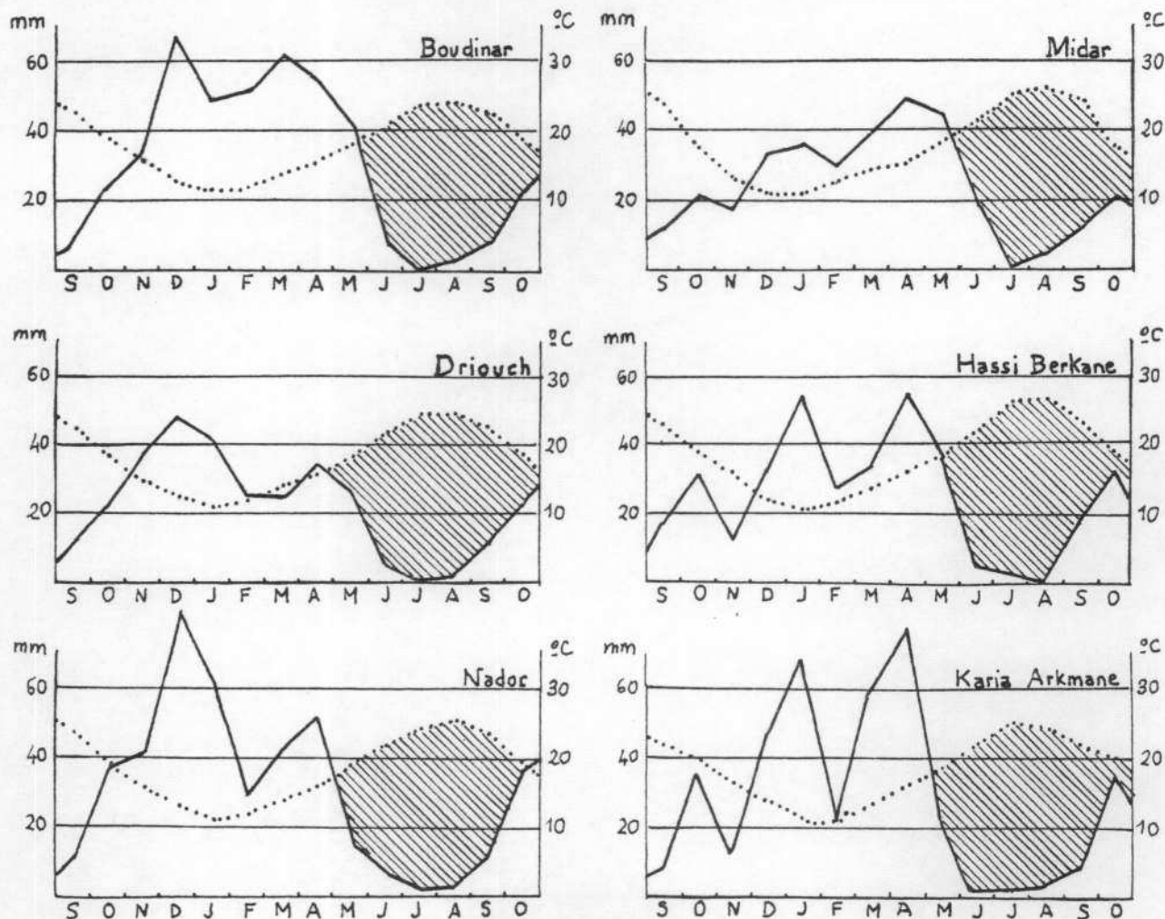
Courbes ombro-thermiques
